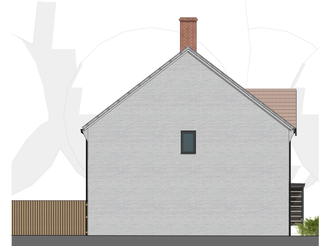
09 SW Elevation 1:100
