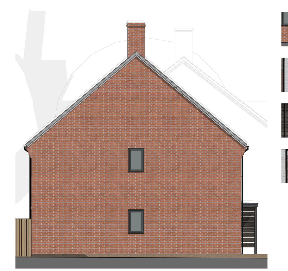
13 SW Elevation 1:100
